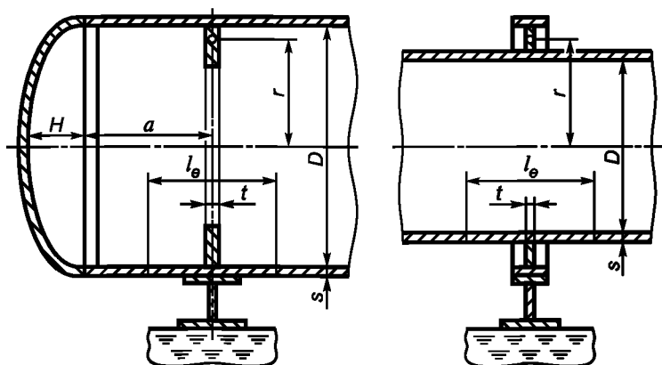
Рисунок 9 — Расчётная схема седловой опоры
