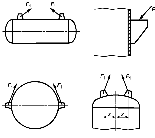
Рисунок 4 — Примеры применения несущих ушек
