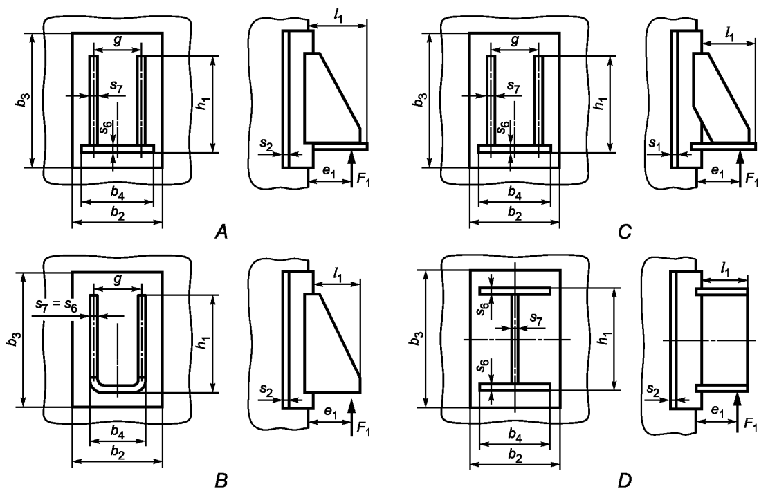
Рисунок 7 — Основные типы опорных лап
