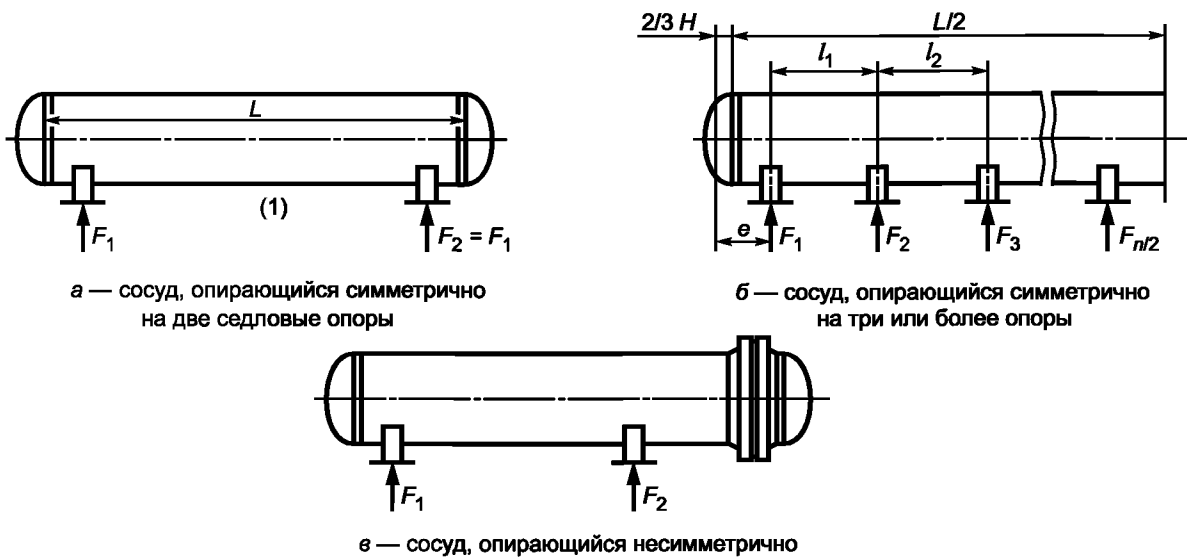
Рисунок 8 — Схемы расположения седловых опор для сосудов аппаратов
