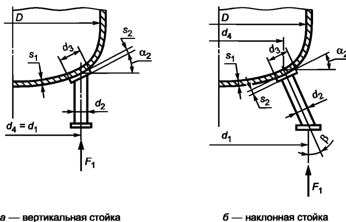
Рисунок 11 — Цилиндрические опорные стойки
