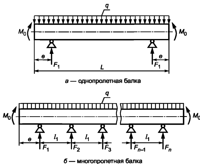
Рисунок 10 — Расчетные схемы эквивалентного сосуда для определения усилий
